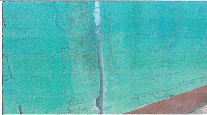
Foto 2: Reparación de muros perimetral de block con tubo ng y malla galvanizadas soleras intermedias y columnas
